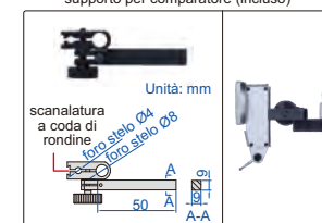
supporto per comparatore (incluso)
