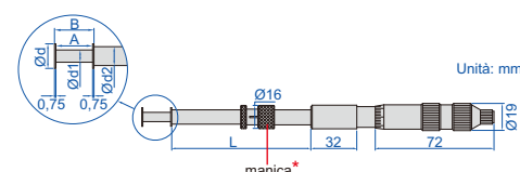
misurare la posizione della scanalatura
