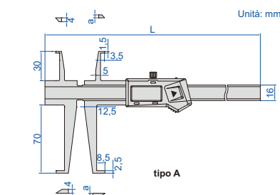
dimensioni da misurare (utilizzare le ganasse superiori)
