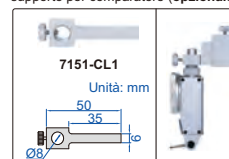
supporto per comparatore (opzionale)
