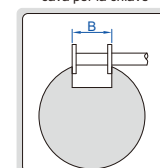
misurare la larghezza della scanalatura
