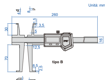
dimensioni da misurare (utilizzare le ganasse inferiori)
