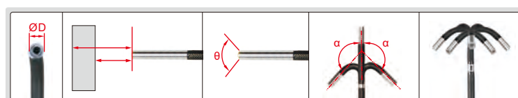
diametro (ØD) profondità di campo (DOF) angolo di campo (θ) campo di curvatura (α) piegare in 4 direzioni
